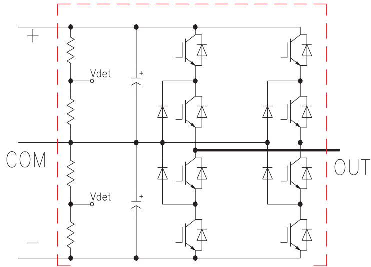
Схема ячейки инвертора с фиксированной нулевой точкой
