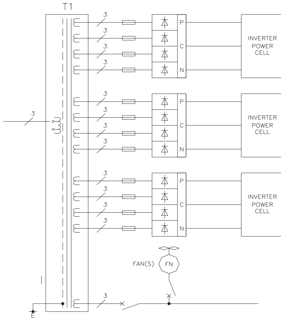
Схема силовой части преобразователя
